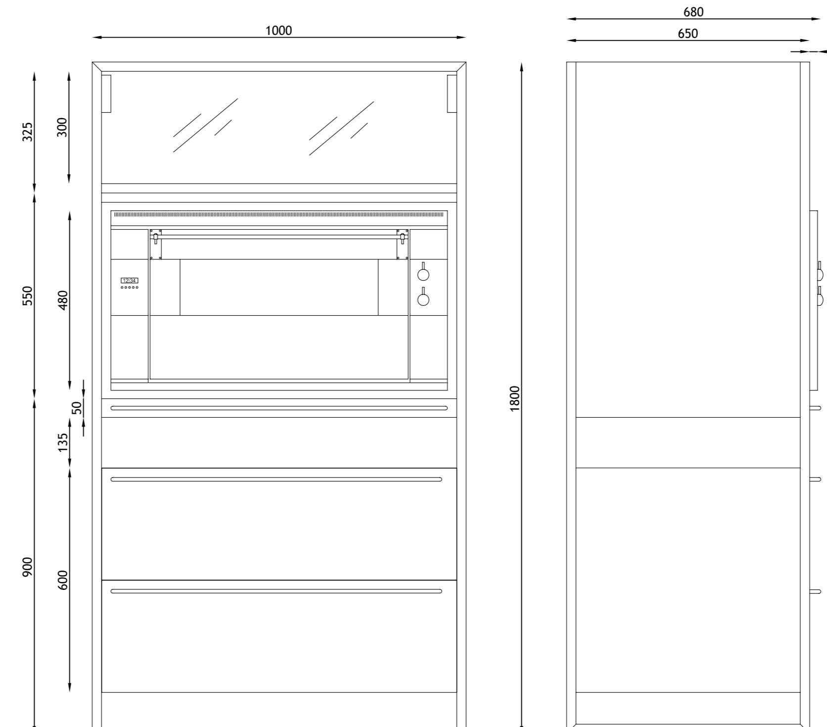
M3-261-000 MÓDUL 100-V/95, (1000x650x1800) CALAIXOS INFERIORS I FORN SMEG S620MMFR 7 (900x480 INDI).
