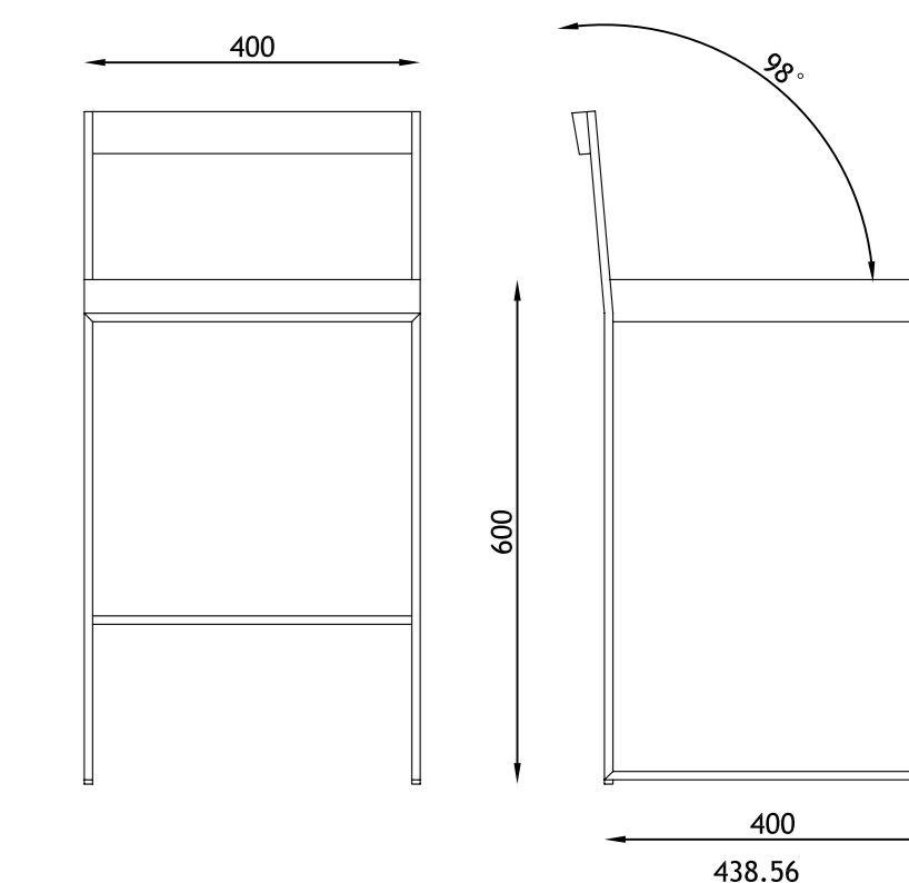
M3-290-000 TABURET SIT-B
