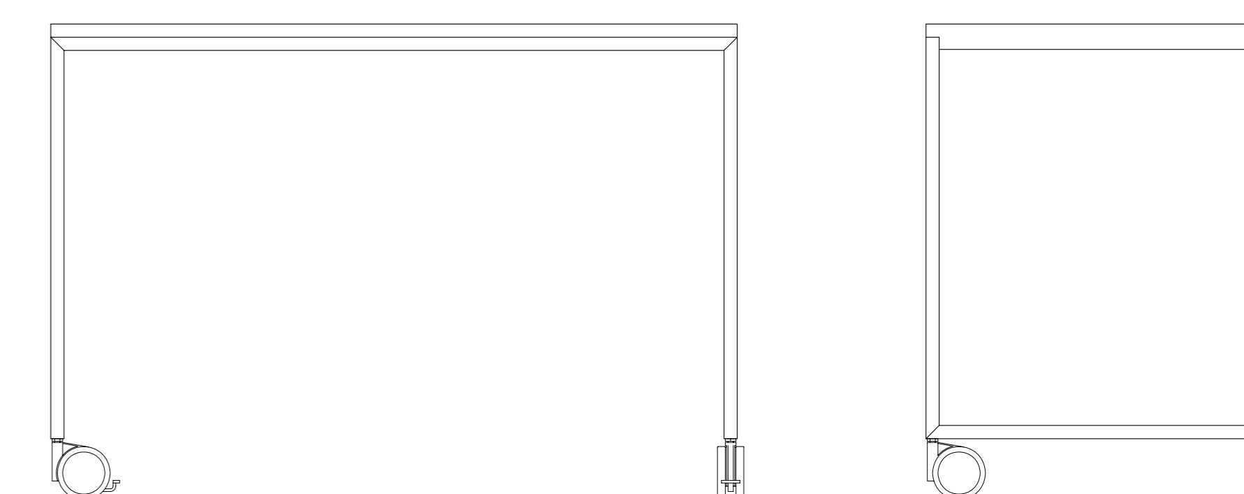
M3-282-000 MÓDUL 100-C/a AMB PLAFÓ ALT (1000x650x1450) SMEG S62645.
