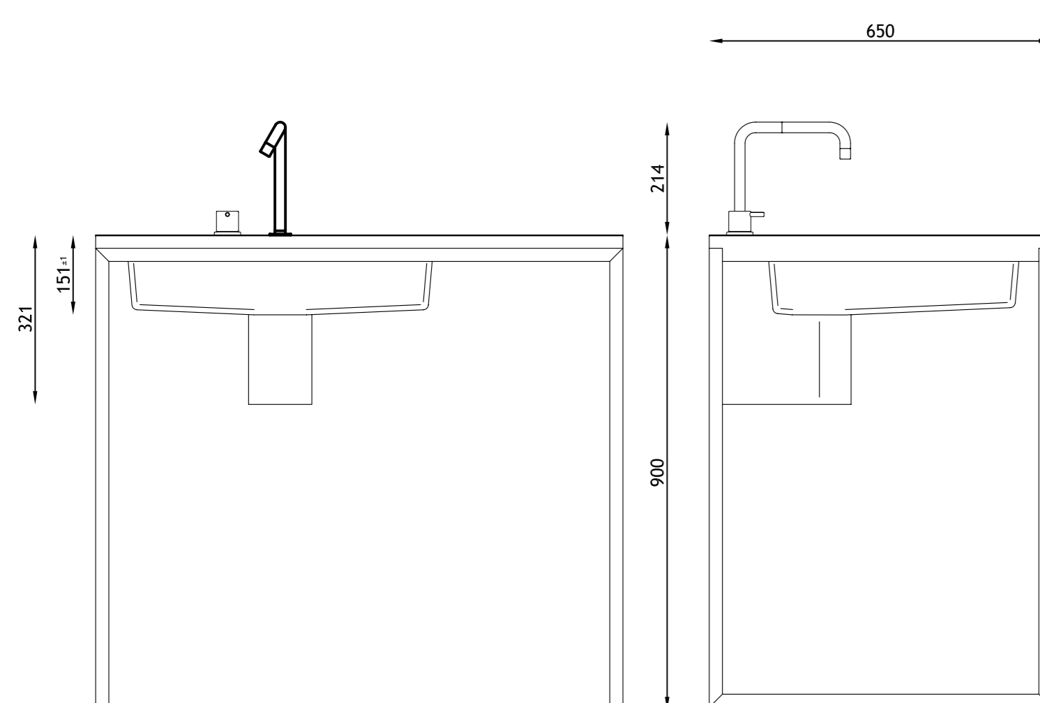
M3-270-000 MÓDUL 100-H (1000x650x900) VOLTA 590.
