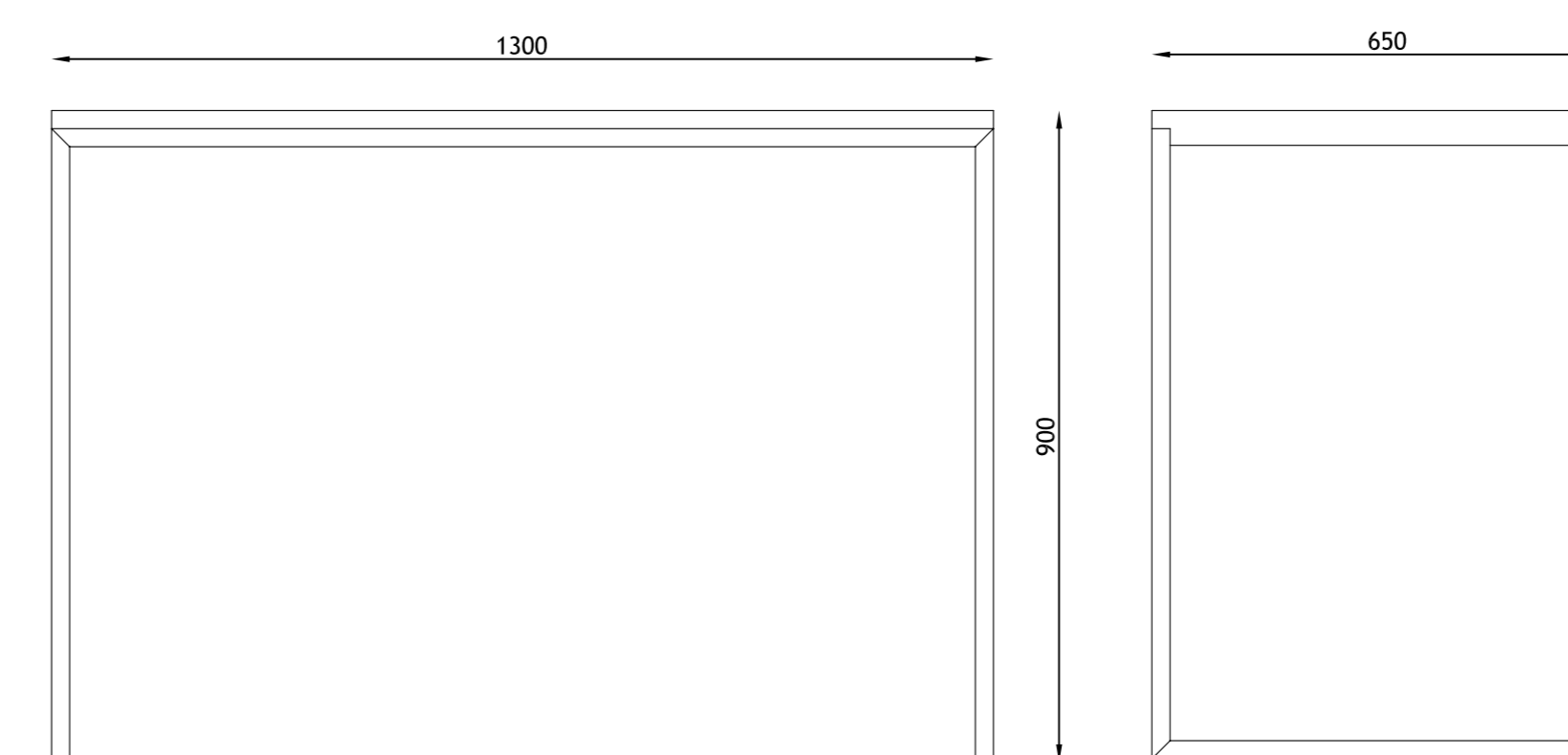
M3-220-000 i M3-222-000 MÓDUL 130 (1300x650x900) 130-R, SOBRE RECICLA (RELACIÓ M3-213-000).
