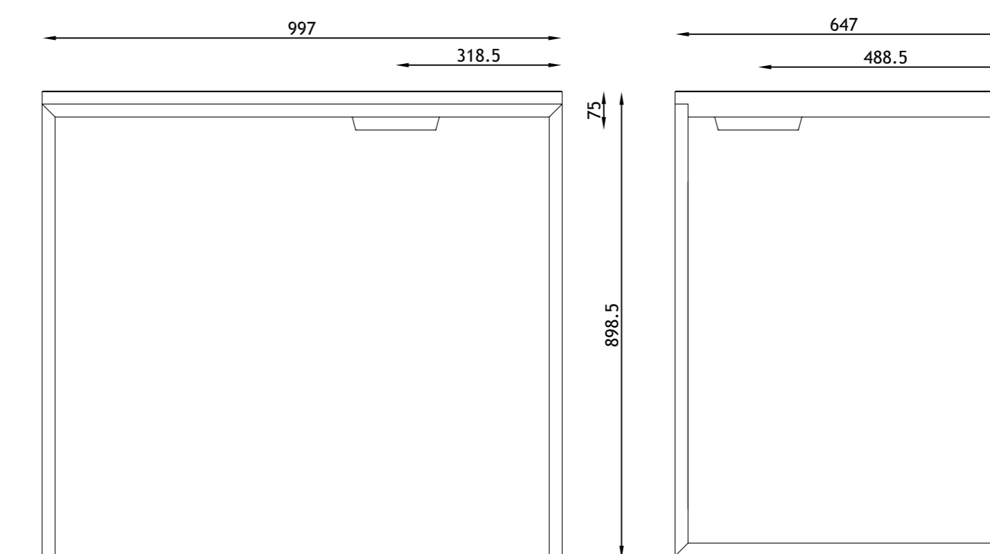
M3-213-000 MÓDUL 100-R (1000x650x900) RECICLA, AMB MÓDUL R (M3-250-000)
