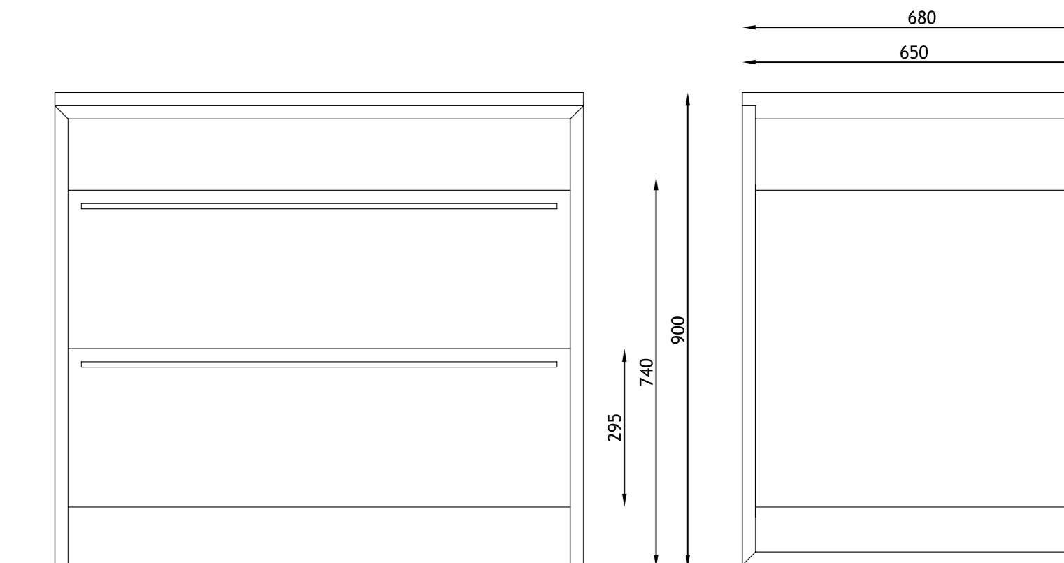
M3-214-000 MÓDUL 100-95 (1000x650x900) CALAIXOS 95.
