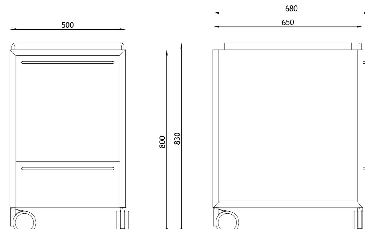
M3-250-000 MÓDUL R (500x650x800) RECICLATGE OGTM ROLL.
