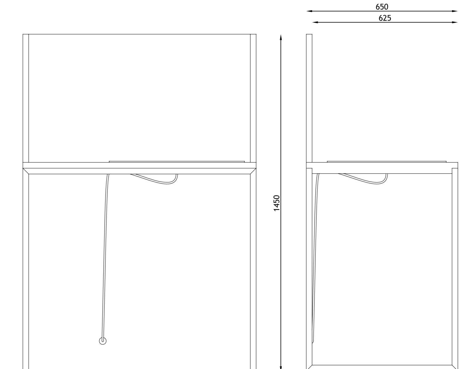
M3-282-000 MÓDUL 100-C/a AMB PLAFÓ ALT (1000x650x1450) SMEG S62645.
