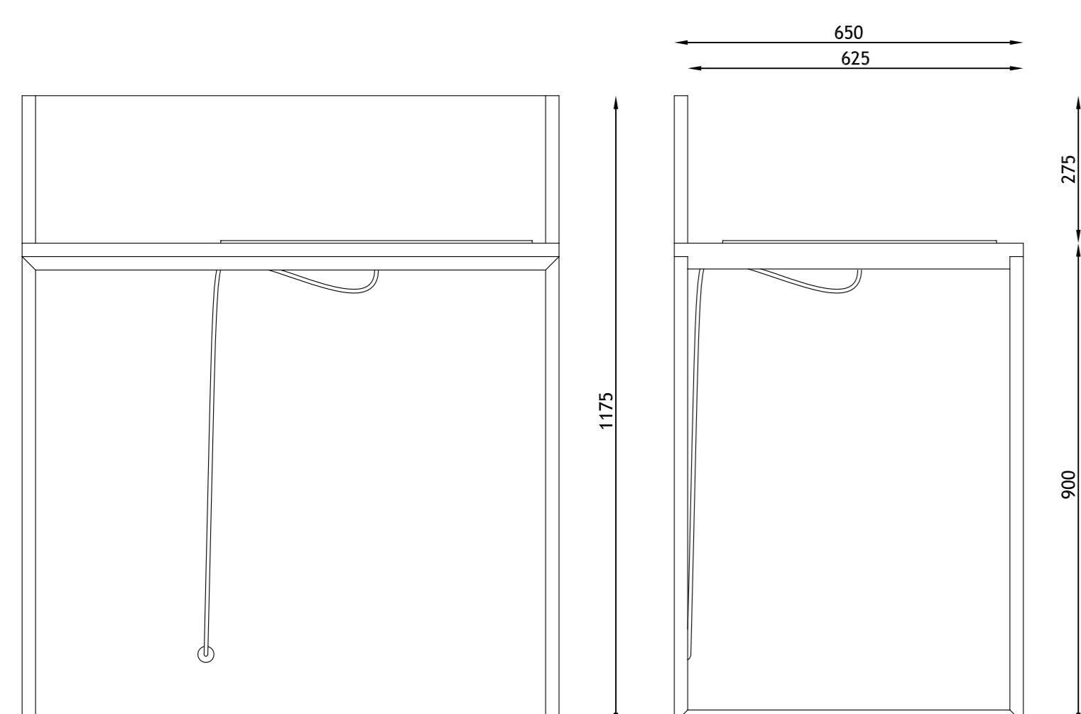
M3-283-000 MÓDUL 100-C/b, AMB PLAFÓ BAIX (1000x650x1175) SMEG S62645.
